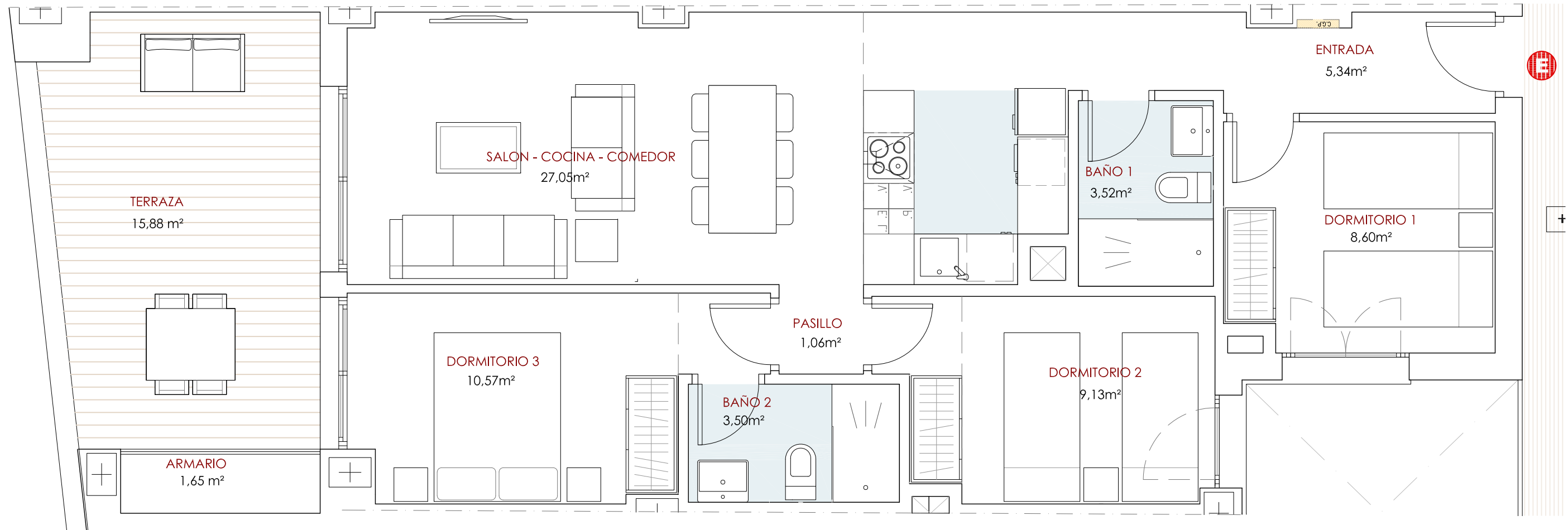
LOCALIZACIÓN PLANTA
