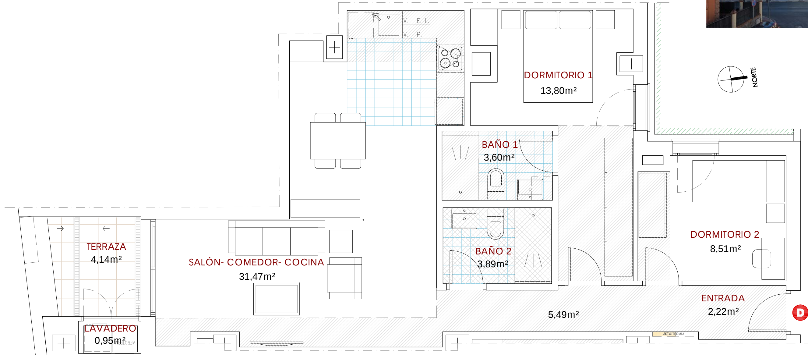
LOCALIZACIÓN PLANTA
